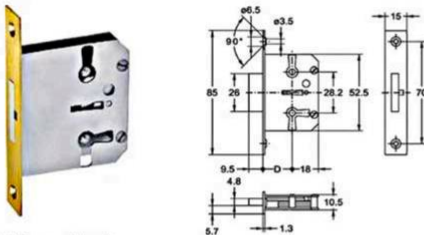
Møbellås 667 (vendbar)
