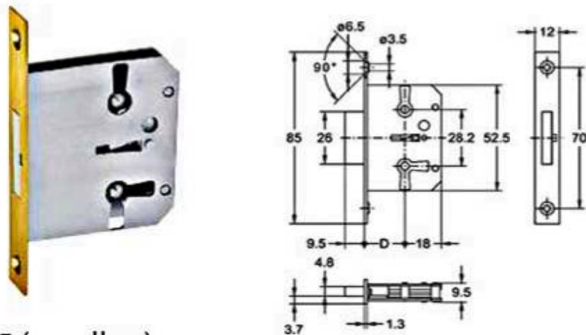
Møbellås 665 (vendbar)
