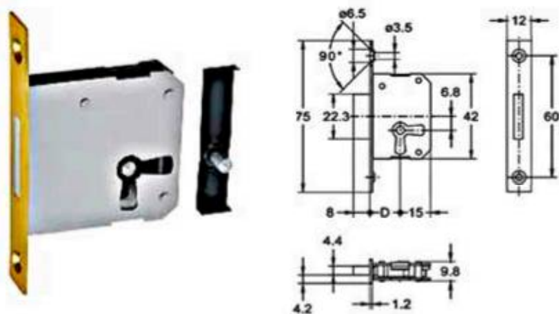
Møbellås 663 (vendbar)
